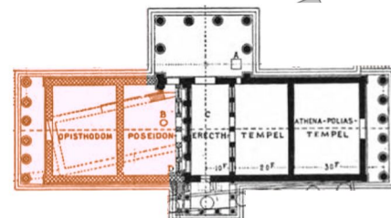
Pełny plan Erechtejonu
